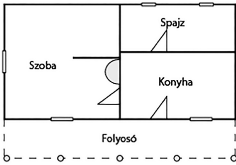
Az egyszobás ház alaprajza, és az eredeti állapotban megmaradt épület Jászladányon a Rácz Aladár utcában
