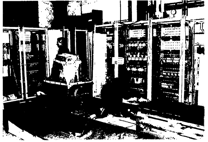
A Perros testhabosító új vezérlőszekrényeit a szerszámüzemben készítik elő.
